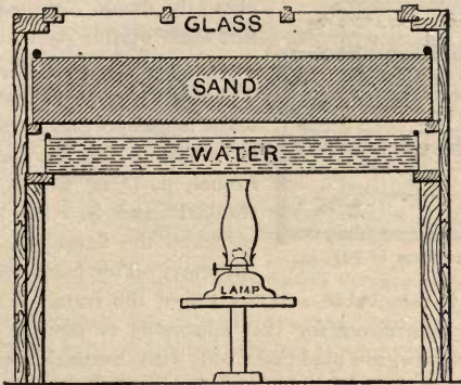
Fig. 33. Simple Propagating-oven.
